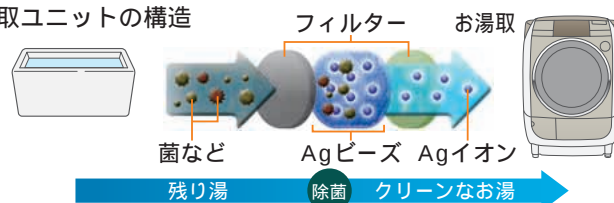
Ag除菌お湯取ユニットの構造
