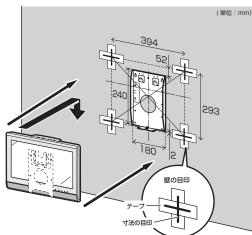
壁掛け金具 AN-130AG1 使用時 (LC-16E5)
