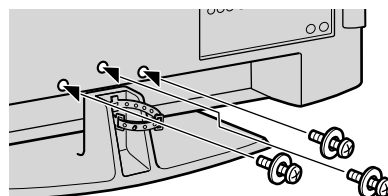
本体固定用ネジ
