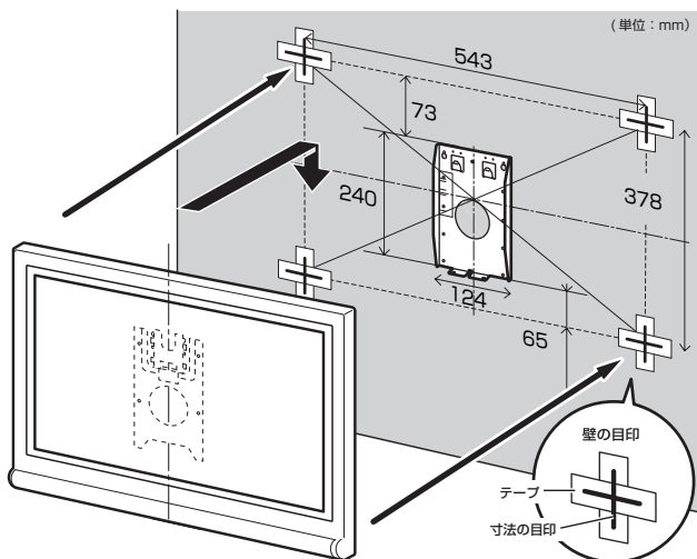
壁掛け金具 AN-130AG1 使用時 LC-22P1 の場合
