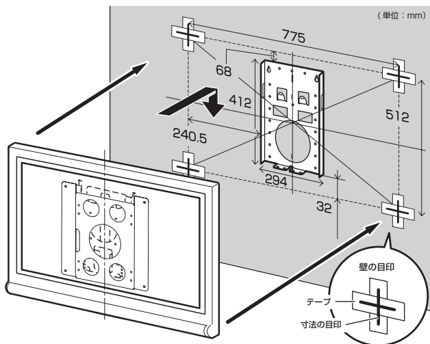
壁掛け金具 AN-37AG2 使用時 LC-32P1 の場合
