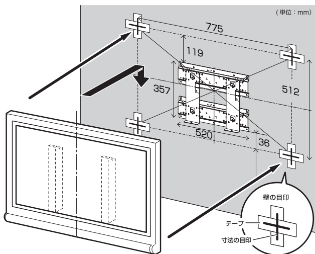
壁掛け金具 AN-37AG4 使用時 LC-32P1 の場合
