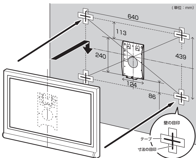
壁掛け金具 AN-130AG1 使用時 LC-26P1 の場合
